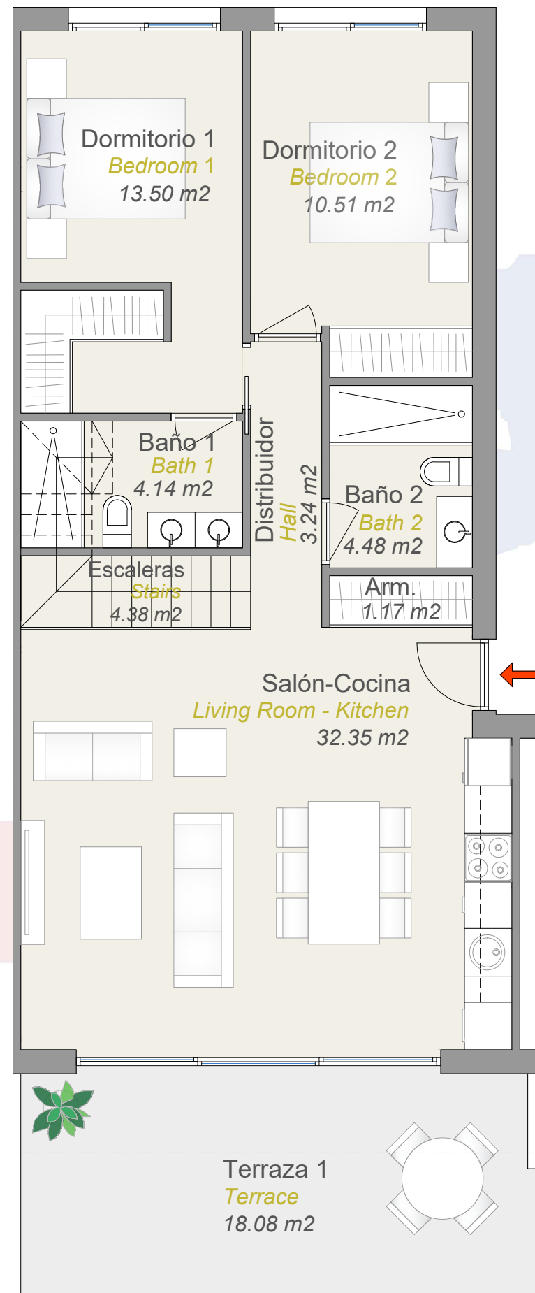
PLANTA PRINCIPAL
